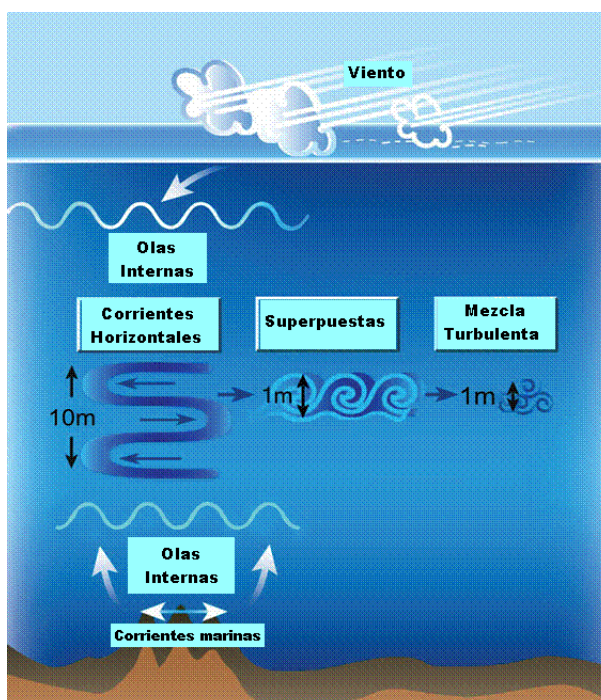
Olas internas y escalas de las mezclas oceánicas. (Del libro: Oceanografía, de Chris Garrett. Véase también: http://www.nature.com/nature/journal/v422/n6931/full/422477a.html )
