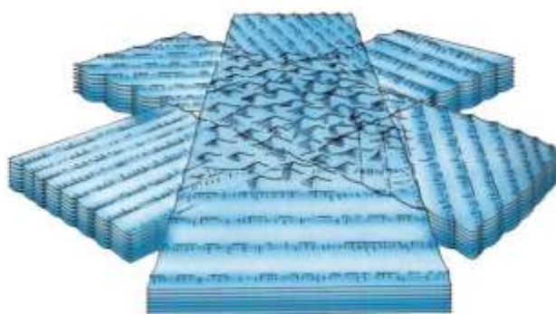
Las olas internas en la interfase entre dos capas de agua de diferentes densidades. Una es más densa (la que está debajo) y la otra es menos densa (la que está arriba). (Del libro: Oceanografía, Gross, p. 204.)
