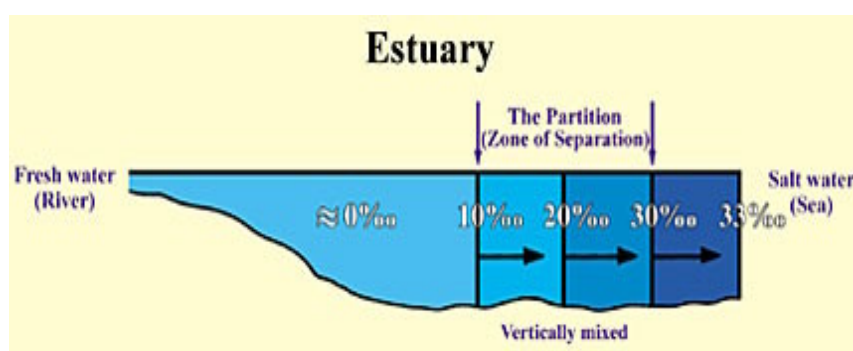
Figur 14: Tværsnit der viser saltholdighed (tusinddele) ved en flodmunding. Vi kan her se opdelingen (opdelingszonen) mellem det ferske og det salte vand. ( Introductory Oceanography , Thurman, s. 301, med mindre ændringer).
