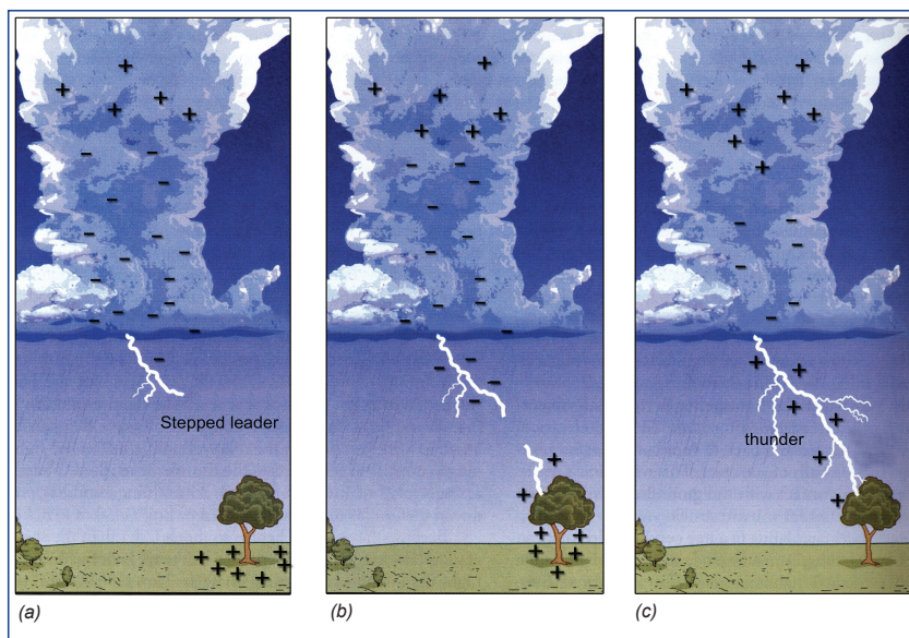
► Model rozvětveného blesku. (a) Záporný náboj koncentrovaný ve spodní části oblaku zesílí natolik, že jej už izolující vrstva vzduchu neudrží a vytvoří se vůdčí výboj blesku mířící k zemi. (b) Vstřícný výboj s kladným nábojem vychází nejčastěji z vyvýšených míst na zemi. (c) Dochází ke spojení záporně nabitého vůdčího a kladně nabitého vstřícného výboje a vzniká mohutný elektrický proud, tzv. hlavní výboj blesku, kterým všechny náboje v oblaku zaniknou.
