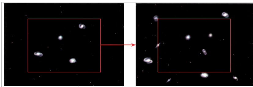
► Tento obrázek ukazuje, že vzdálenost mezi galaxiemi či kupami galaxií se neustále zvětšuje a že vesmír se tedy rozpíná.
