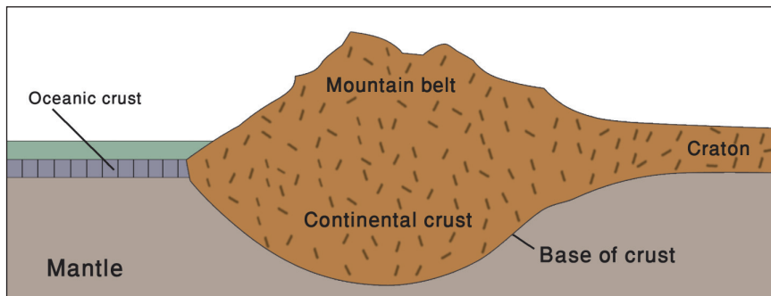
► Obrázek znázorňuje "kořeny" hor. Některé tyto kořeny mohou zasahovat šedesát kilometrů hluboko do země.
